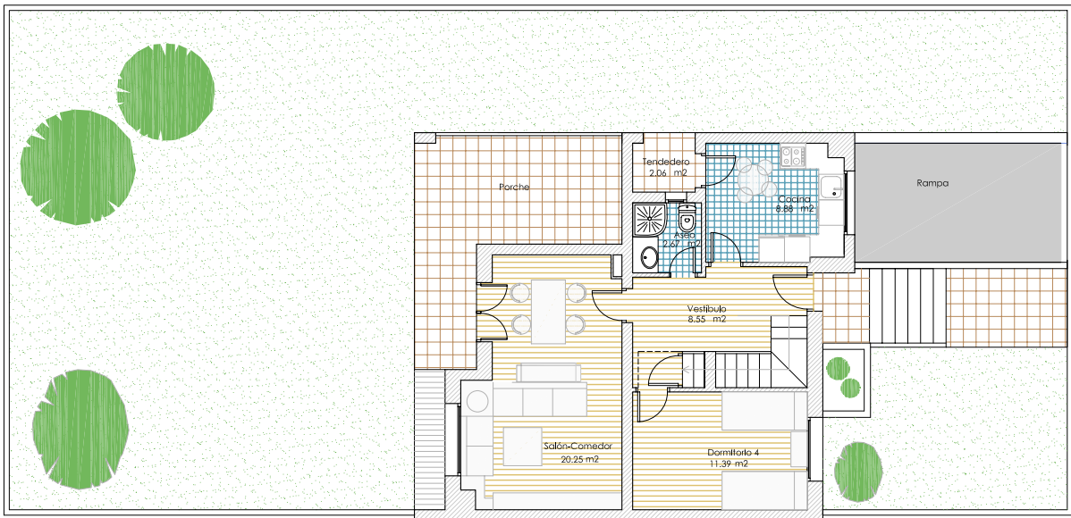
PLANTA BAJA
