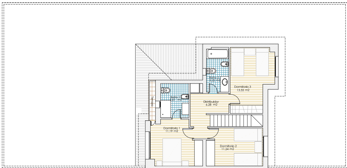
PLANTA PRIMERA
