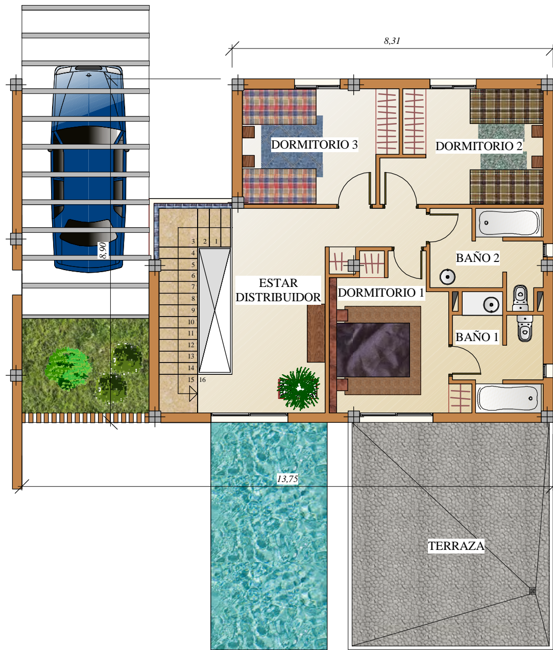
PLANTA PRIMERA
